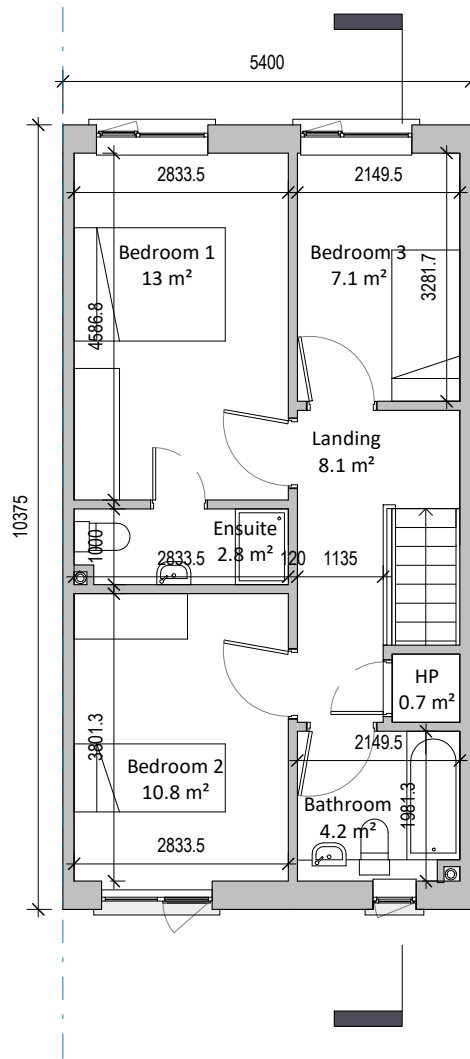
② Type 2 Level 01 1:100
